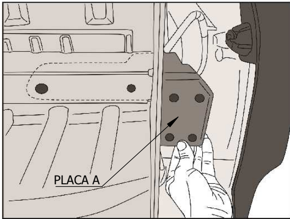
A2 - VISTA INFERIOR LADO CONDUCTOR
